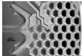
Rückenmarkregenerationsimplantat
