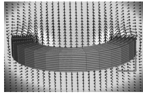
Magnetfeld einer Spule berechnet mit CONCEPT-II.
